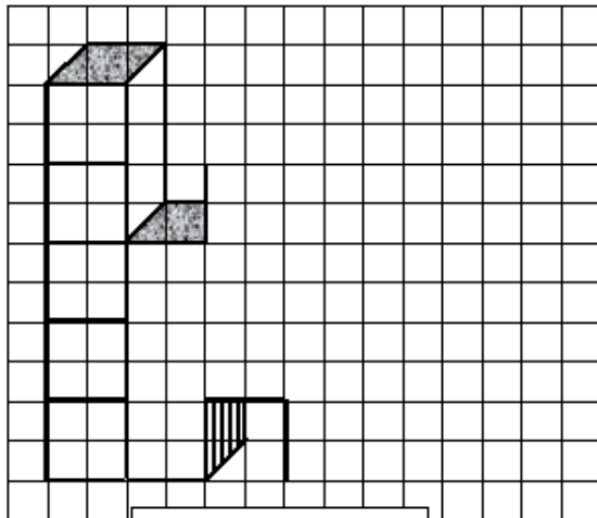
Vue Nord-Ouest
